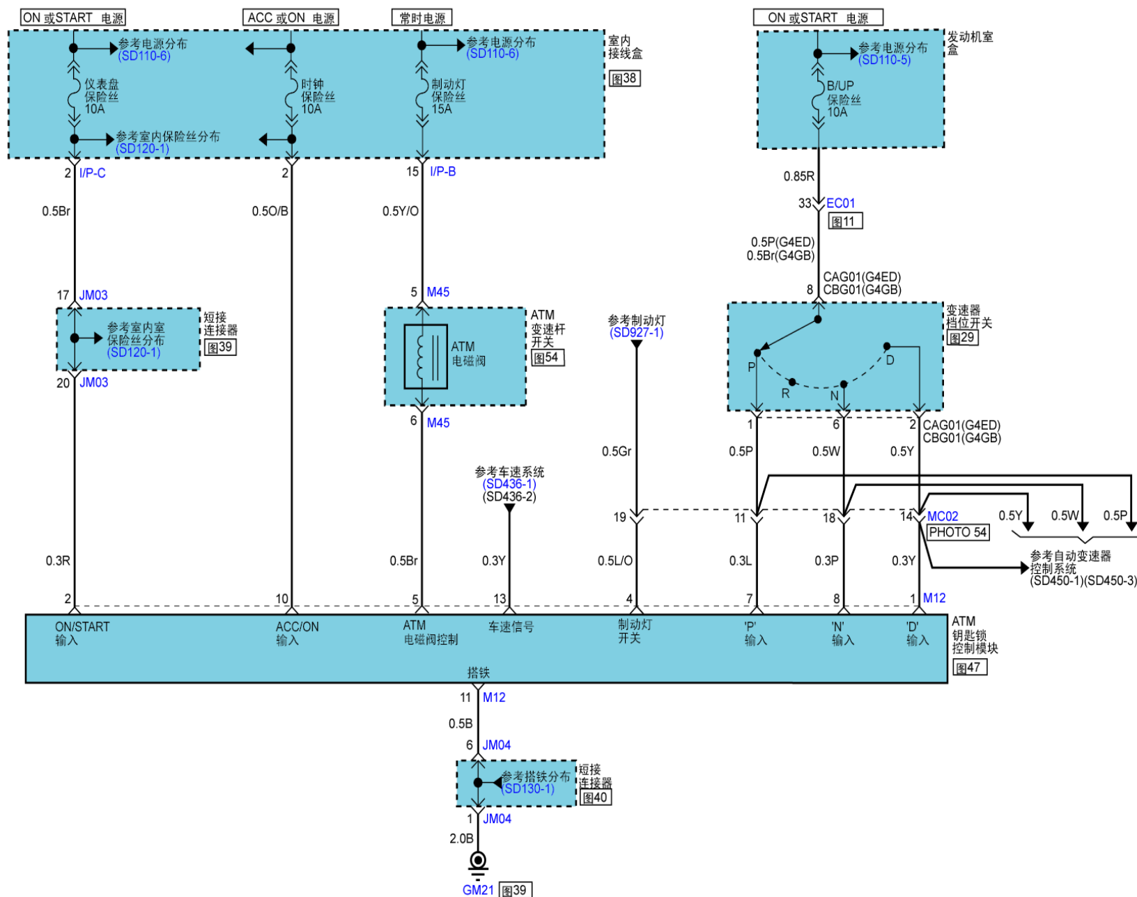
变速杆锁系统(1)
